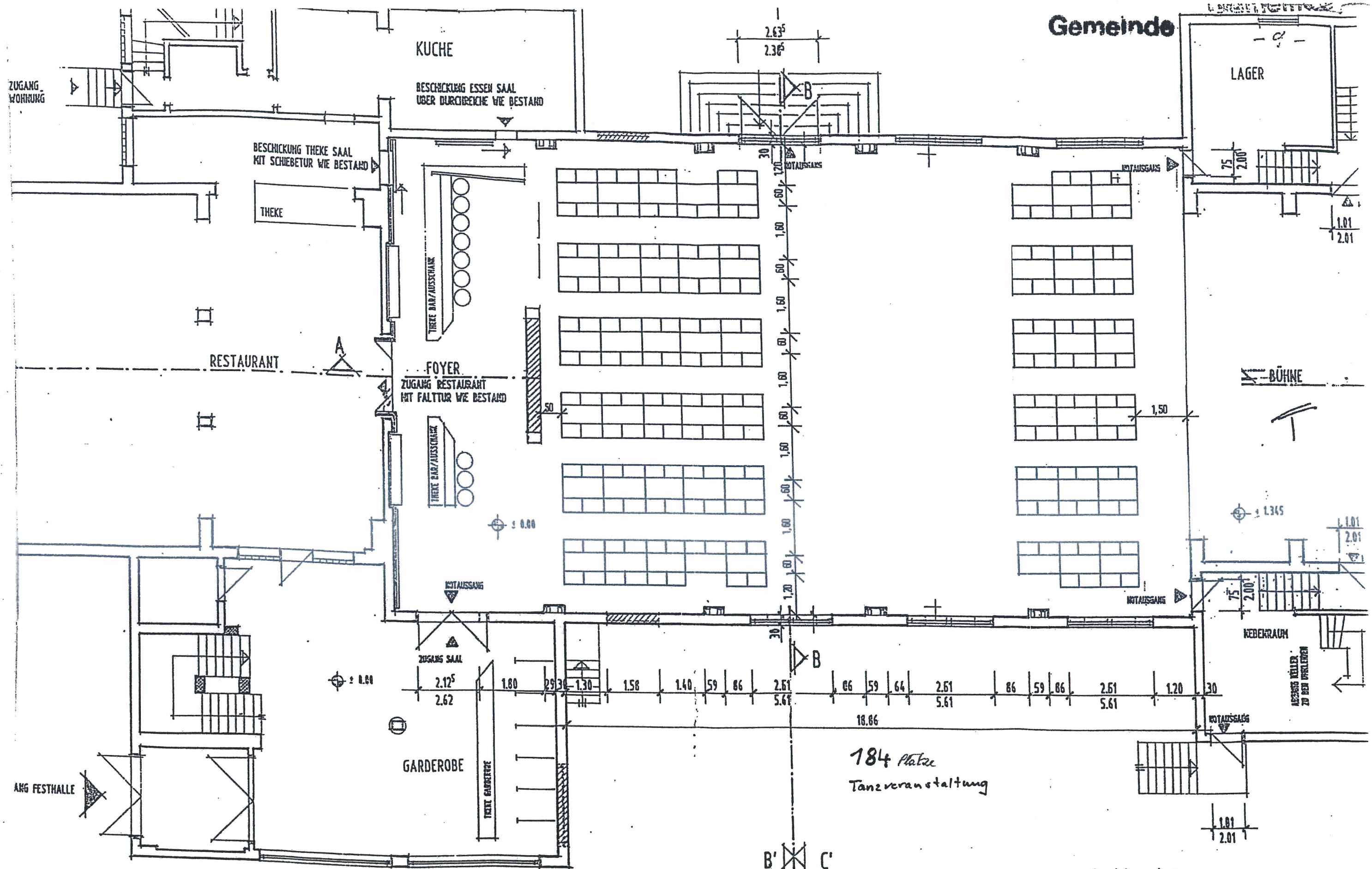
UNDRISS EG BESTUHLUNGSPLAN HALLLE BOBENHEIM-ROXHEIM
